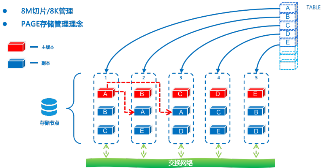
图 3-1 多副本存储
