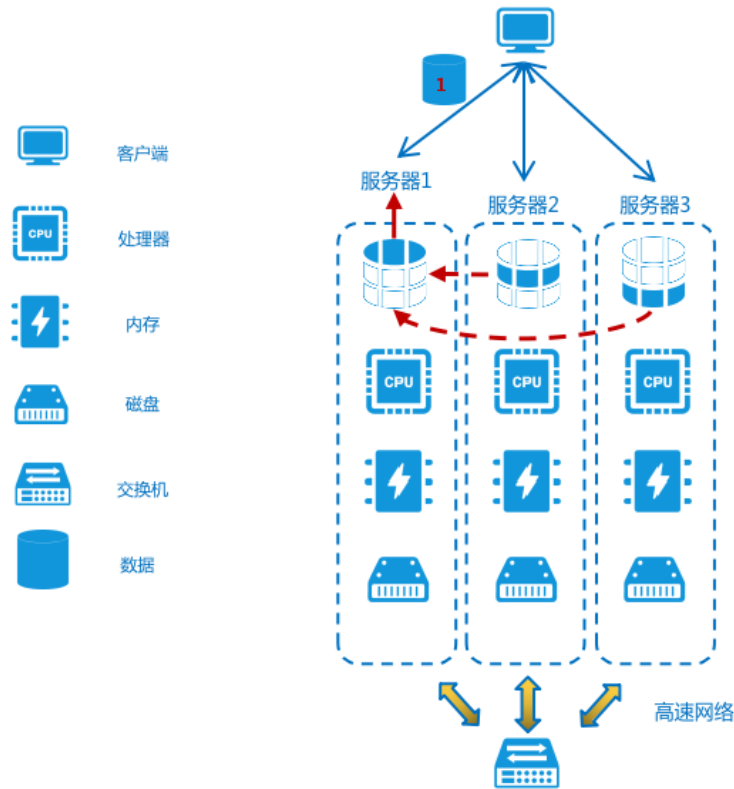
图 2-2 无共享架构
